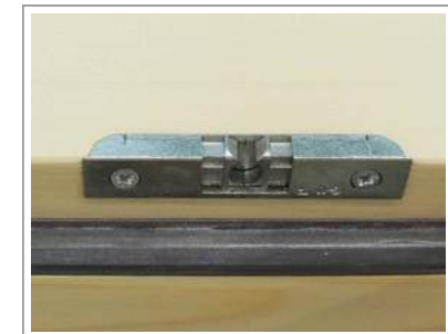
SCHNÄPPER Halter optional mit ETÖ, AV4D, EAV4, EAV4+ Schloss Oben montiert!
